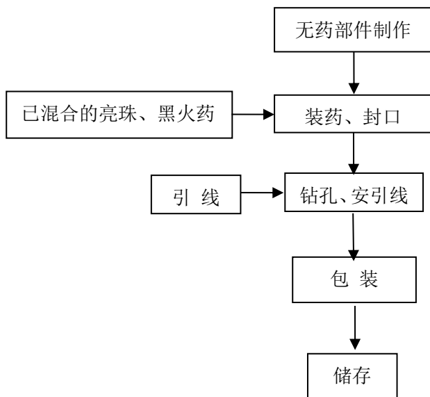
图 2.4-6 喷花类产品生产工艺流程图
