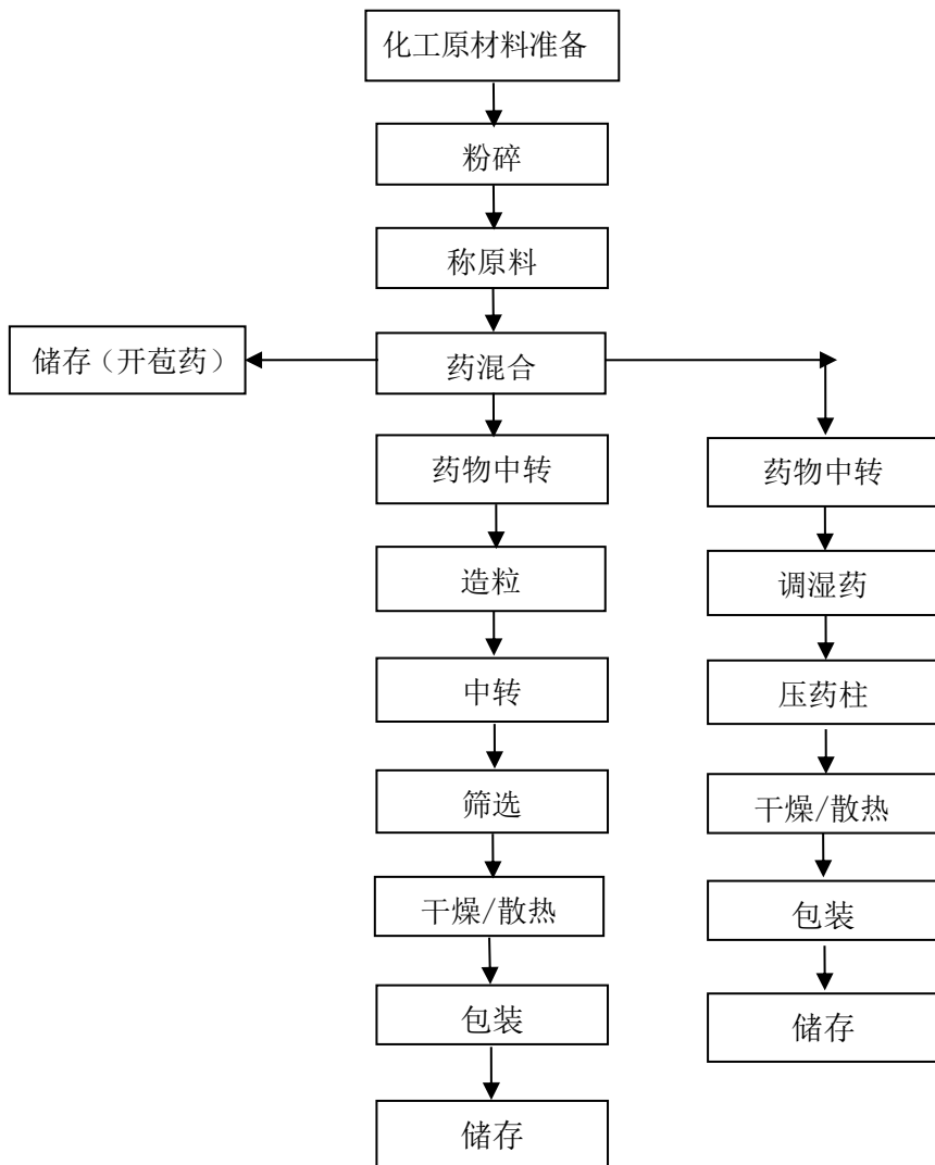
图 2.4-1 药物裸药效果件（亮珠、药柱、开苞药）生产工艺流程图
