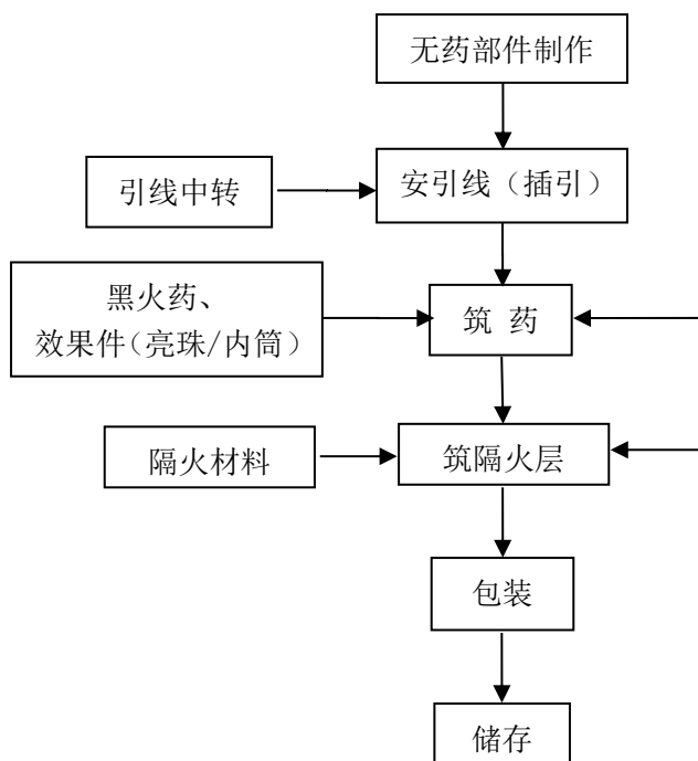
图 2.4-5 吐珠类产品生产工艺流程图
