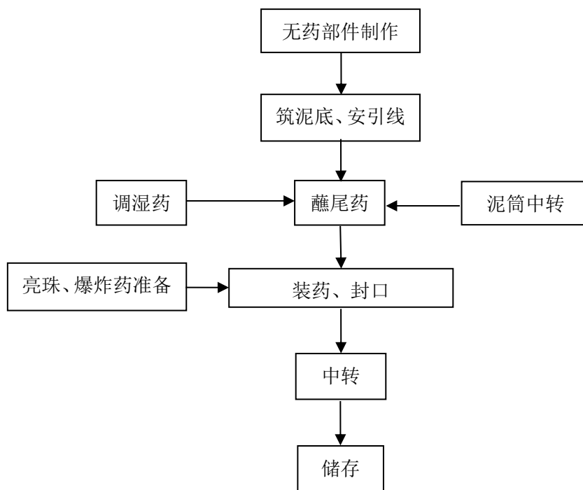
图 2.4-3 效果件内筒（机械装内筒）生产工艺流程图
